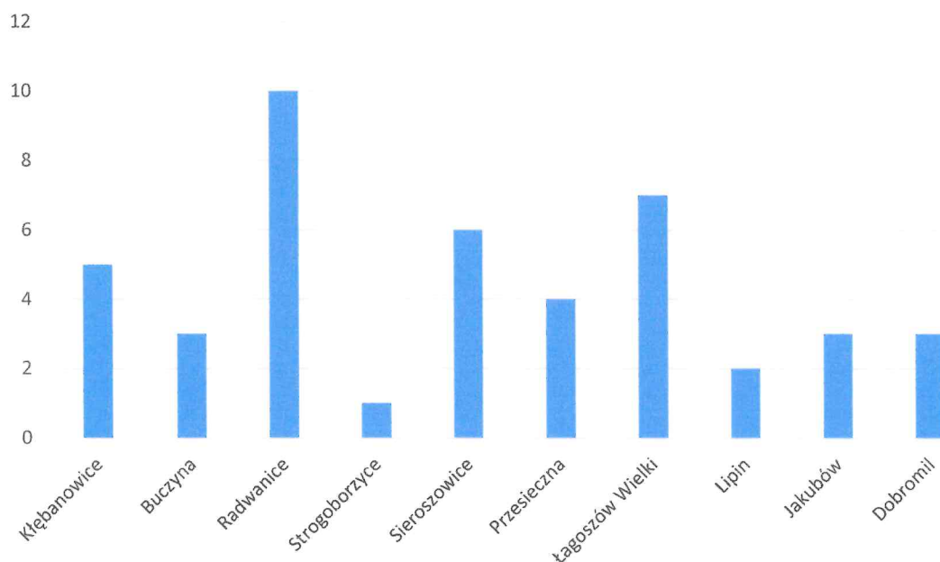
Wykres nr 1. Ilość przepompowni w Gminie Radwanice.
