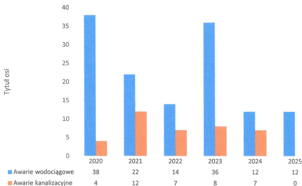
Wykres 5. Ilość awarii wodociągowych i kanalizacyjnych w latach 202-2025.
